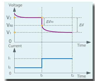
DCIR Test
