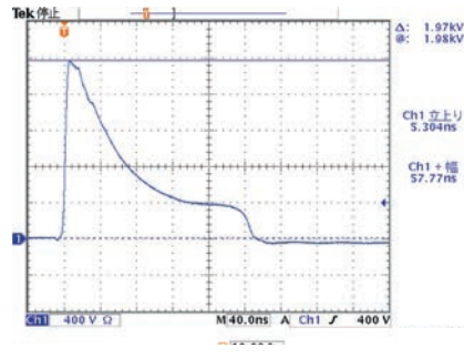
EUT LINE OUTPUT waveform : 50 Ω
